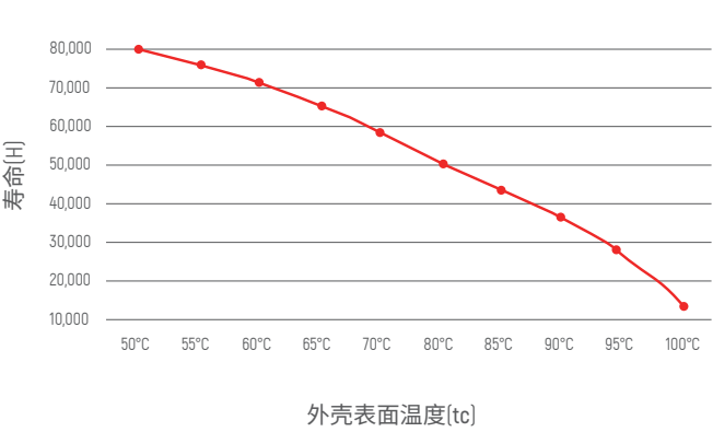
寿命 vs tc温度
