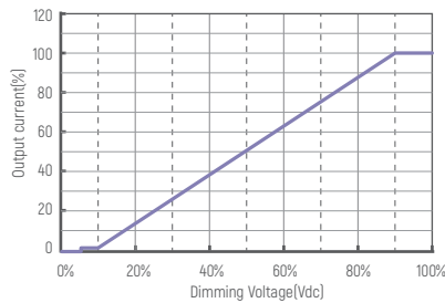
PWM曲线
