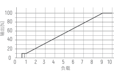
调光曲线
