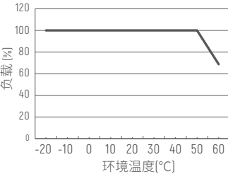
降额曲线
