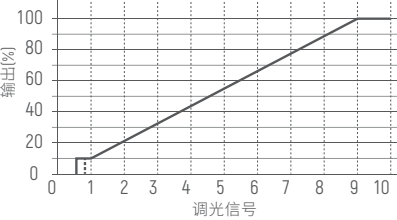
调光曲线
